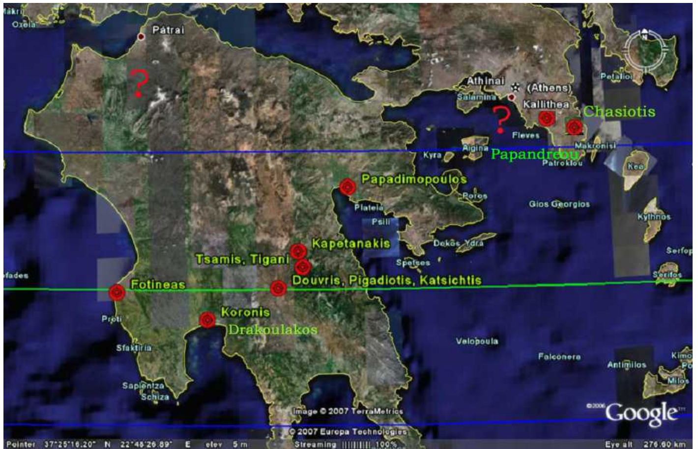
Σχ 8: Διασπορά παρατηρητών κατά την επικείμενη επιπρόσθηση του αστεροειδούς 694-Ekard.
