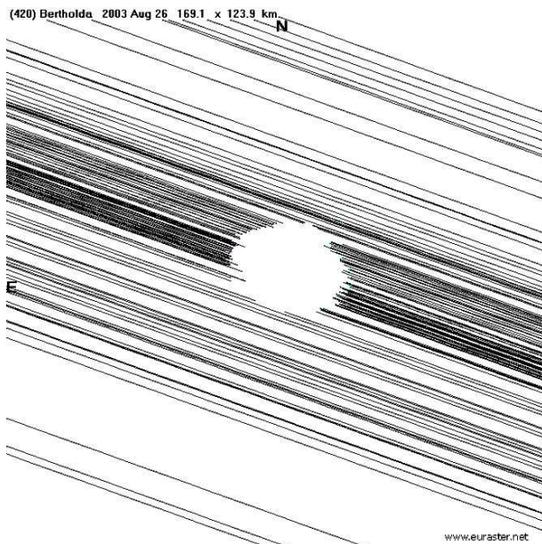
Σχ 4: Το σχήμα και οι διαστάσεις του αστεροειδούς υπολογίζονται με μεγάλη ακρίβεια από τους χρόνους καταγραφής της απόκρυψης για κάθε παρατηρητή, ανάλογα με τις γεωγραφικές του συντεταγμένες.
