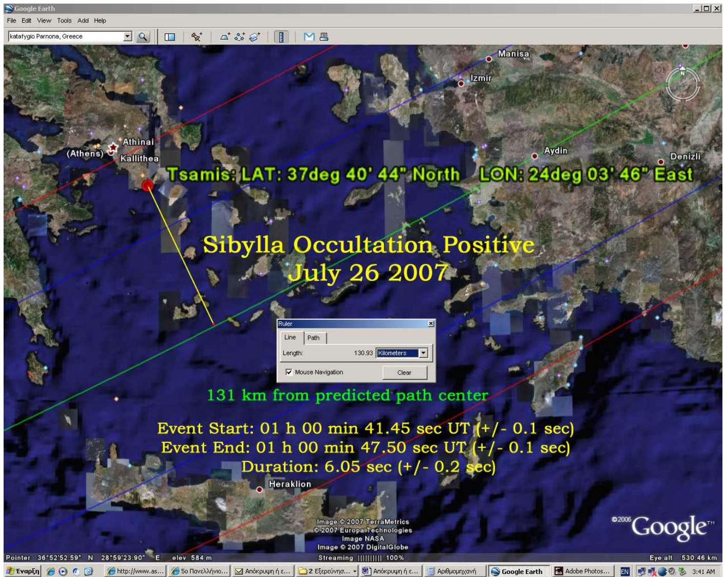
Σχ 11: Απόκλιση του προβλεπόμενου από το πραγματικό μονοπάτι. Από τη θέση παρατήρησης, παρ' όλο που απείχε 131 χλμ από το προβλεπόμενο κέντρο, είχαμε σχεδόν τη μέγιστη δυνατή διάρκεια απόκρυψης (6.05 sec.) Υποθέτουμε ότι η απόκλιση της πρόβλεψης πλησιάζει τα 130 χλμ.
