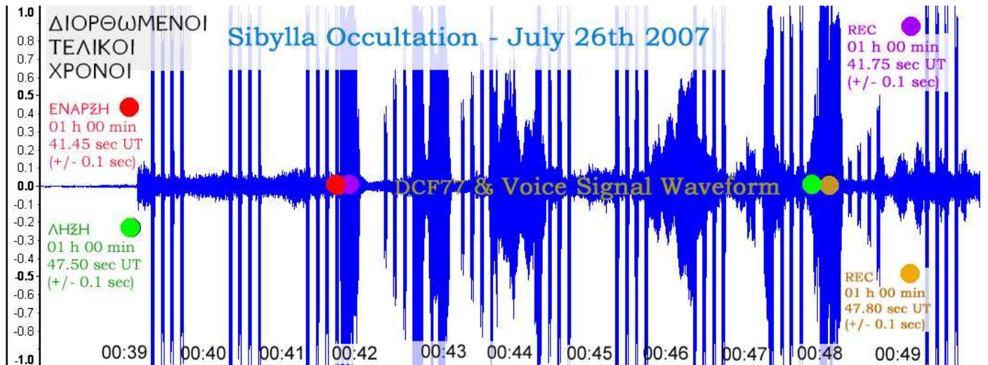
Σχ 10: Κυματομορφή του ήχου που εγγράψαμε κατά την παρατήρηση της επιπρόσθησης του Αστεροειδής Sibylla. Πέμπτη, 26 Ιουλίου 2007, νότια του Λαυρίου και ώρα: UT 01:00:41.55 - UT 01:00:47.50
